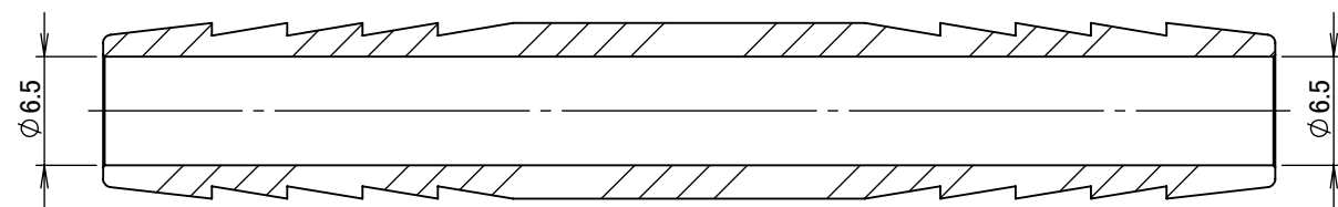
断面図 A-A
