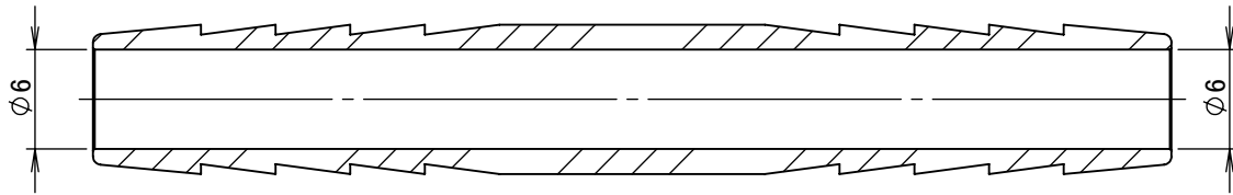
断面図 A-A
