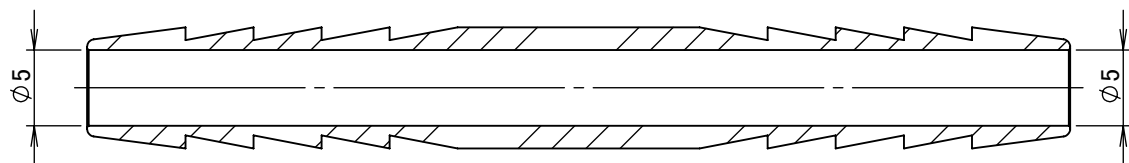
断面図 A-A
