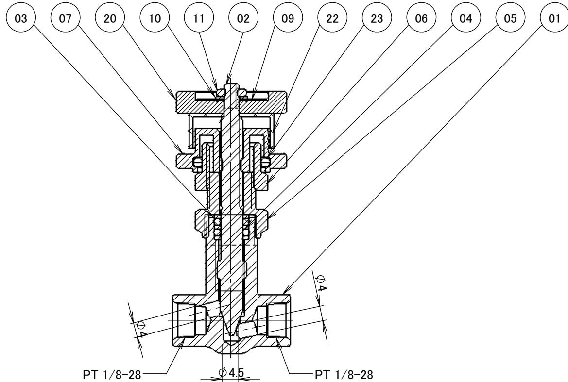
断面図 A-A
