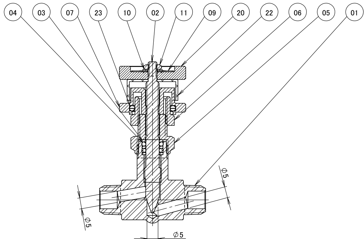
断面図 A-A
