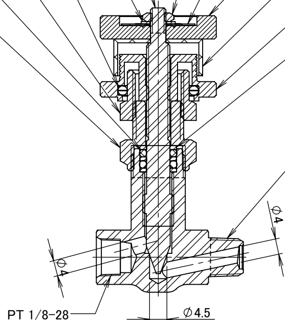
断面図 A-A
