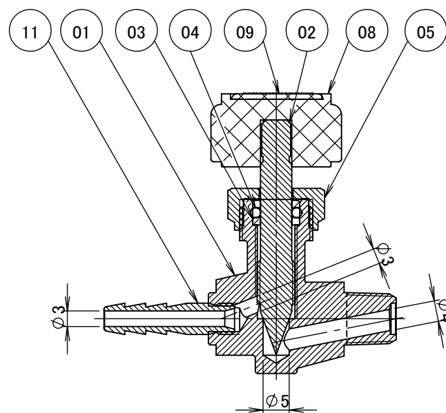
断面図 A-A
