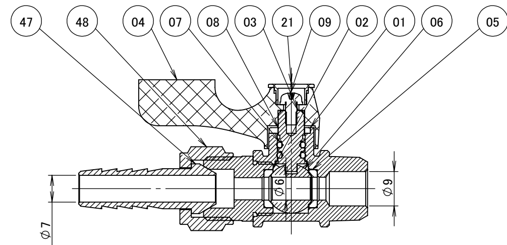
断面図 A-A
