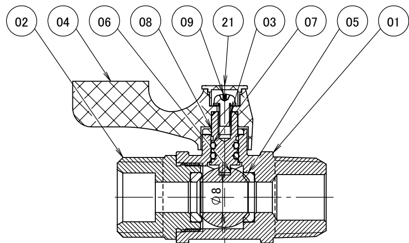
断面図 A-A
