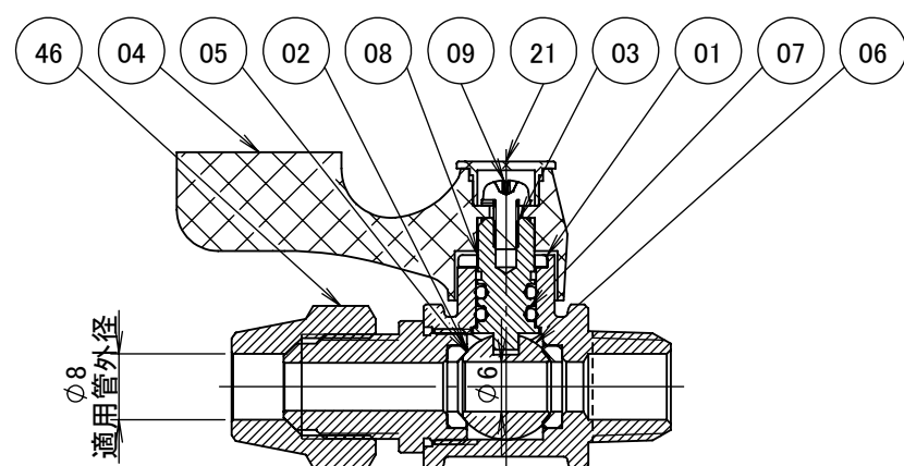
断面図 A-A
