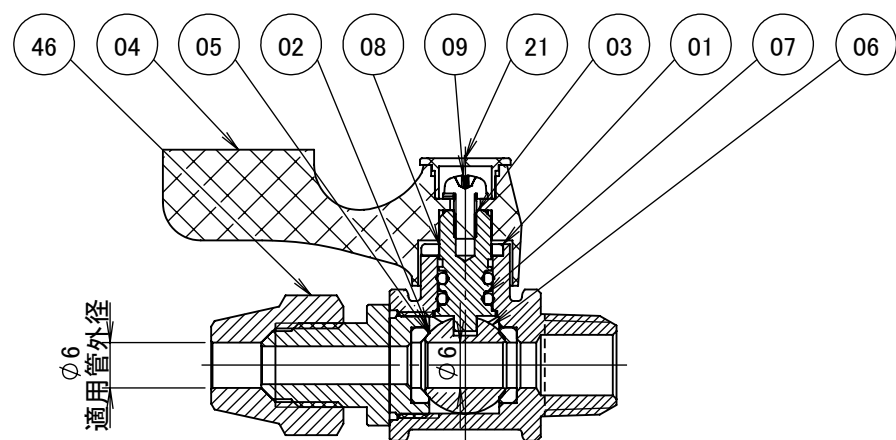
断面図 A-A
