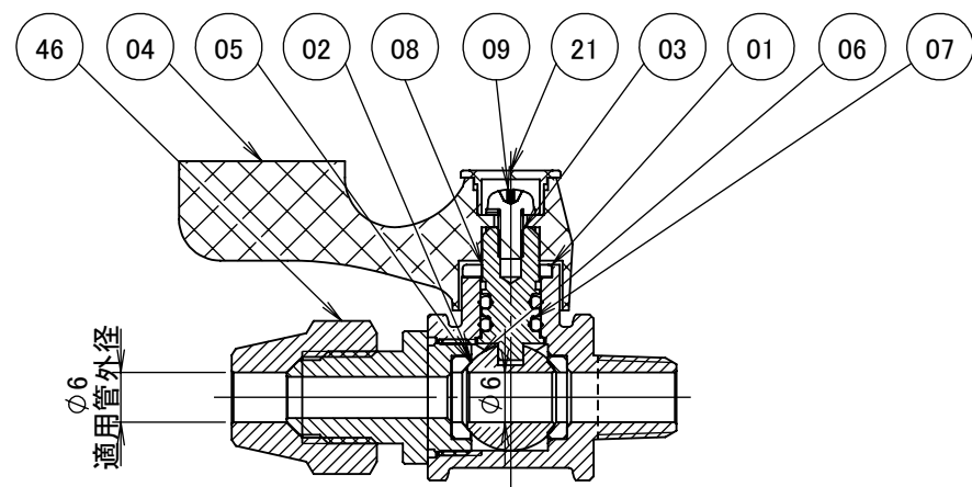
断面図 A-A
