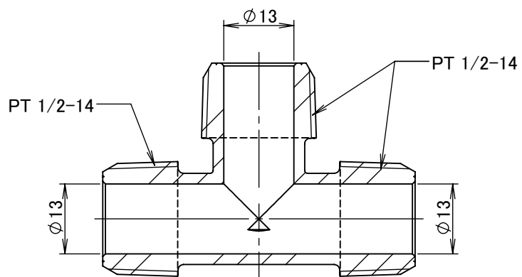
断面図 A-A
