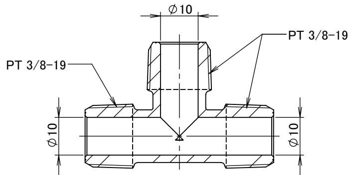
断面図 A-A
