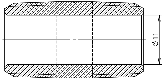
断面図 A-A
