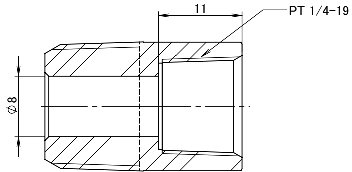
断面図 A-A
