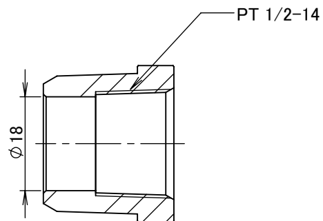
断面図 A-A
