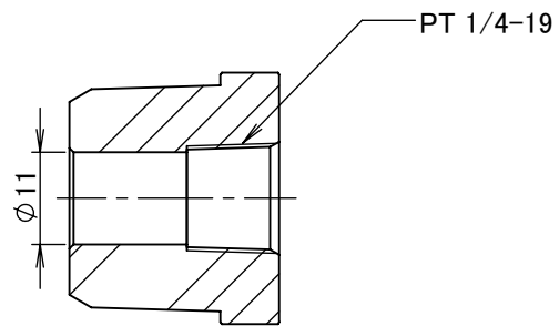
断面図 A-A
