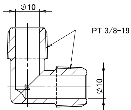
断面図 A-A
