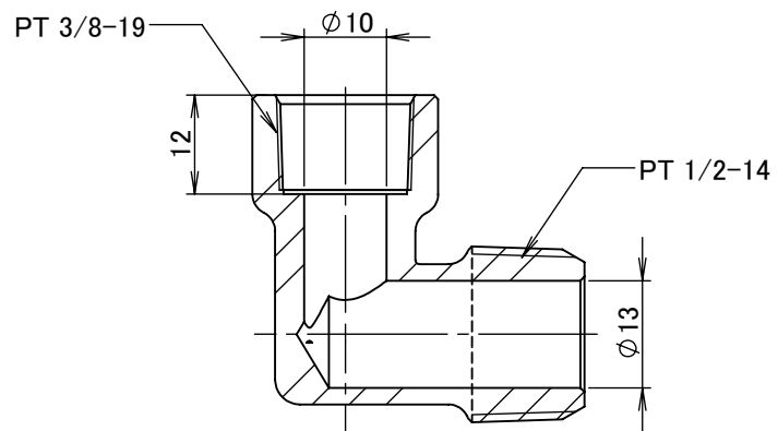
断面図 A-A
