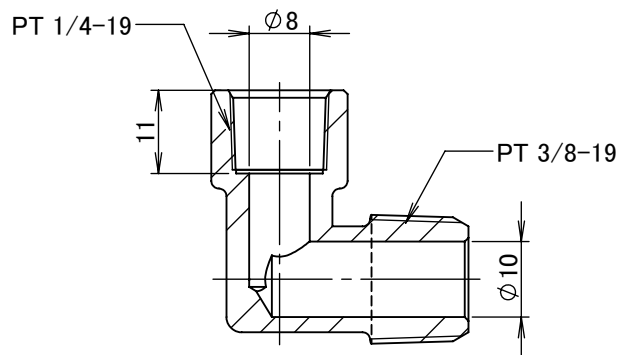
断面図 A-A
