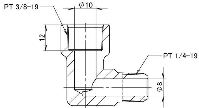
断面図 A-A
