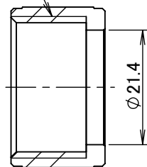
断面図 A-A
