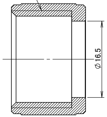
断面図 A-A
