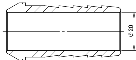
断面図 A-A
