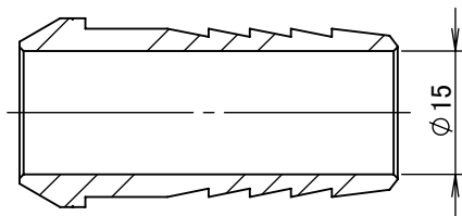
断面図 A-A
