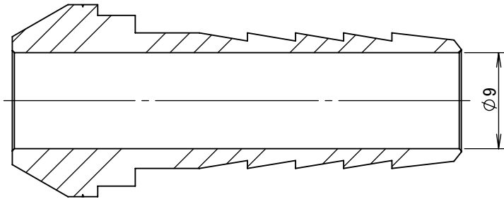
断面図 A-A
