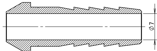
断面図 A-A
