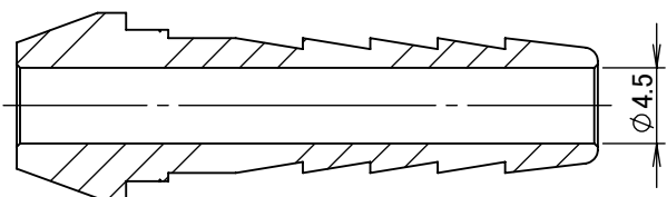
断面図 A-A
