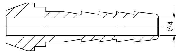
断面図 A-A
