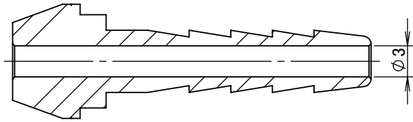
断面図 A-A
