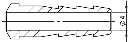
断面図 A-A
