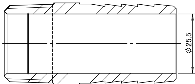
断面図 A-A
