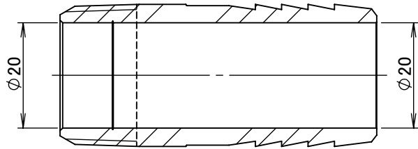
断面図 A-A
