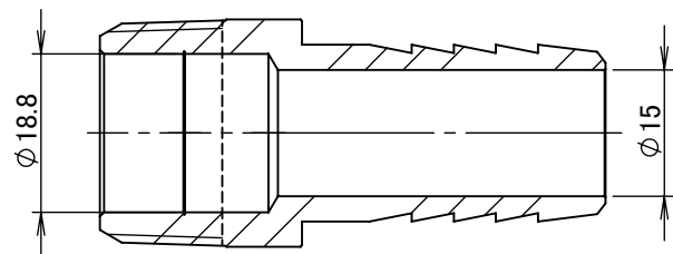
断面図 A-A
