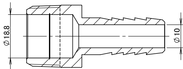
断面図 A-A
