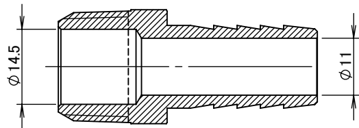
断面図 A-A
