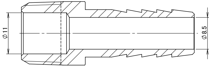
断面図 A-A
