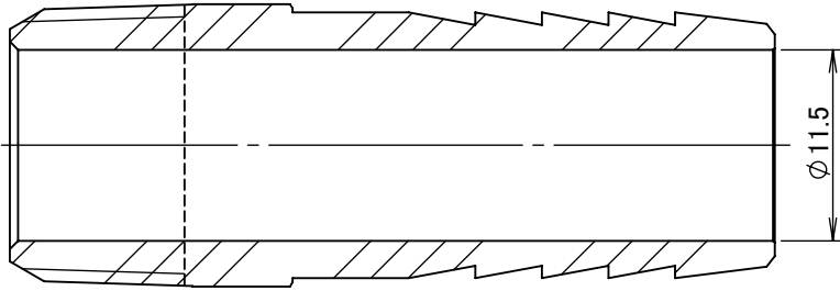
断面図 A-A
