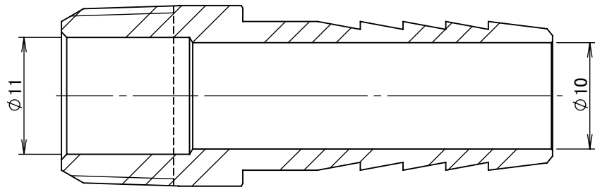
断面図 A-A
