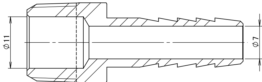
断面図 A-A
