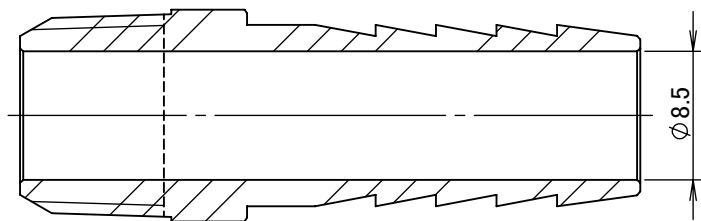
断面図 A-A
