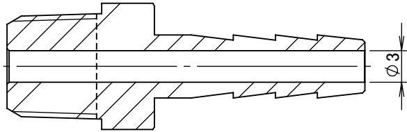
断面図 A-A
