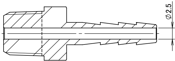
断面図 A-A
