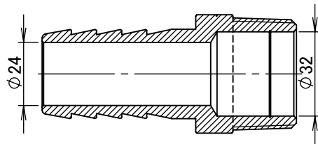
断面図 A-A
