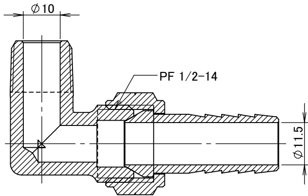
断面図 A-A
