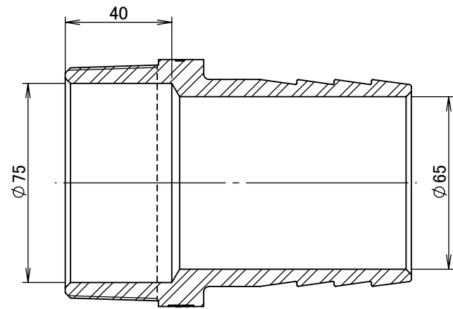
断面図 A-A
